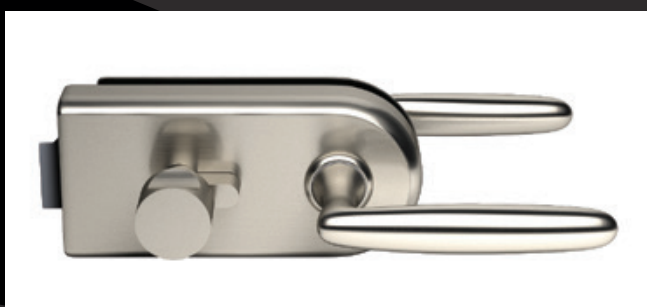
Zamek: Rotonda z blokadą WC , Klamka: Omega Kolor: Stal nierdzewna szczotkowana
