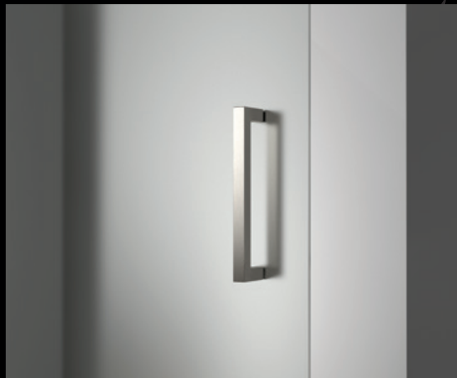
Pochwyt / Pullhandle / Stossgriff: PW4.3 Długość / Length / Länge: 30 cm Profil kwadratowy / Square profile / Viereckprofil: 2.5 cm x 2.5 cm
